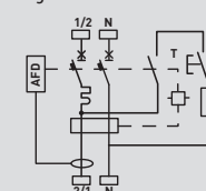
Magnetotermico differenziale
