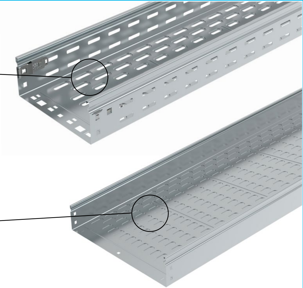
Passerella forata imbutita
